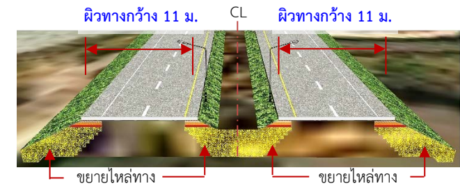
รูปที่ 2 แสดงรูปตัดทางหลวง เกาะกลางแบบกดเป็นร่อง
